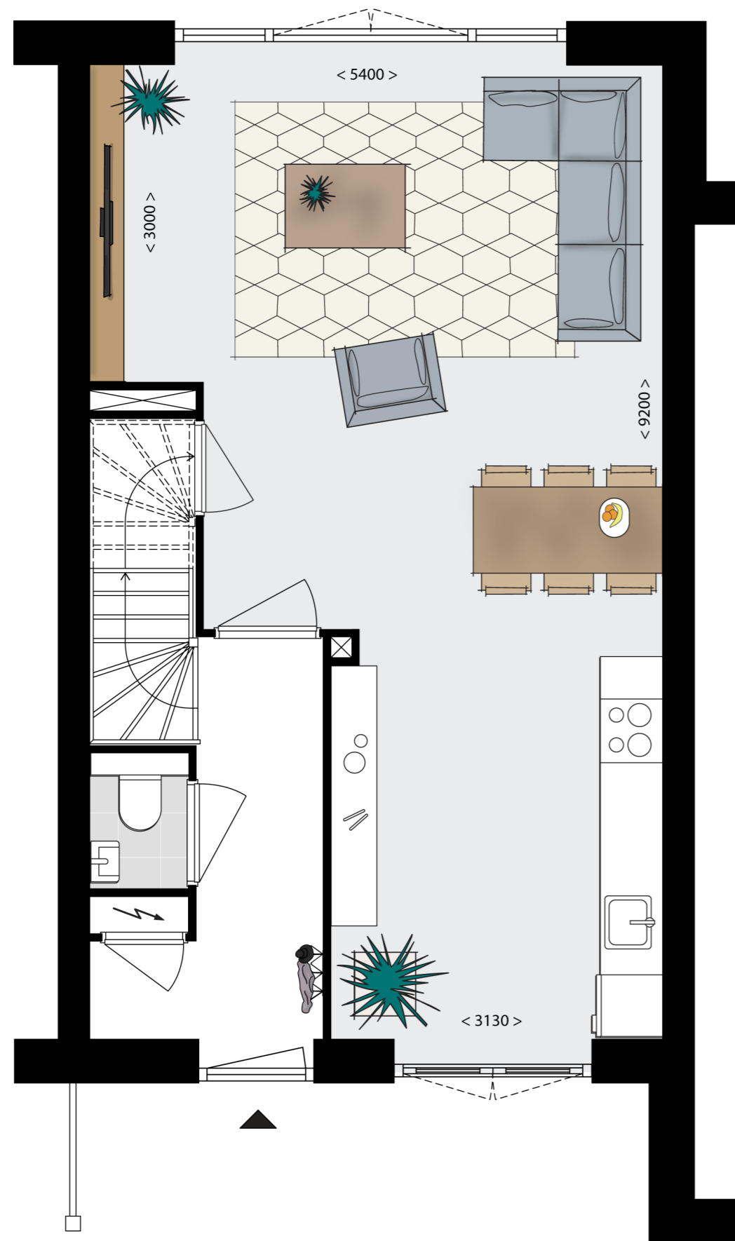
begane grond
